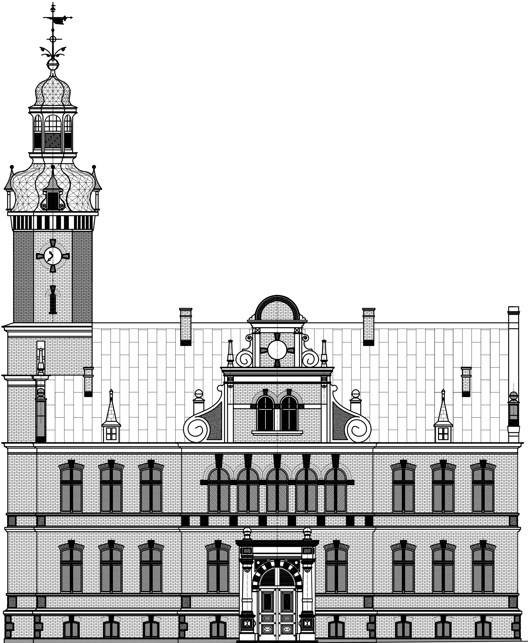
ELEWACJA ZACHODNIA - SKALA 1:100
