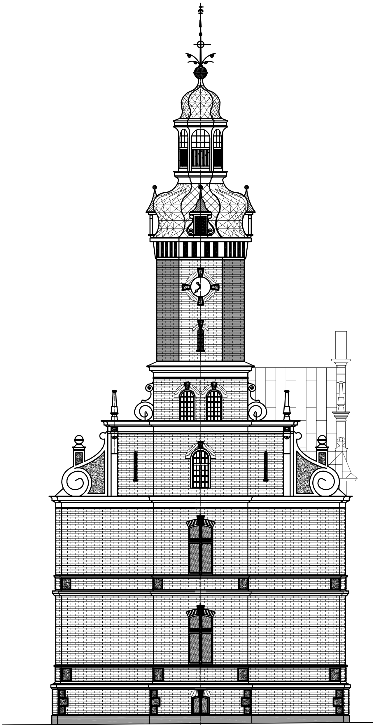
ELEWACJA PÓŁNOCNA - SKALA 1:100.
