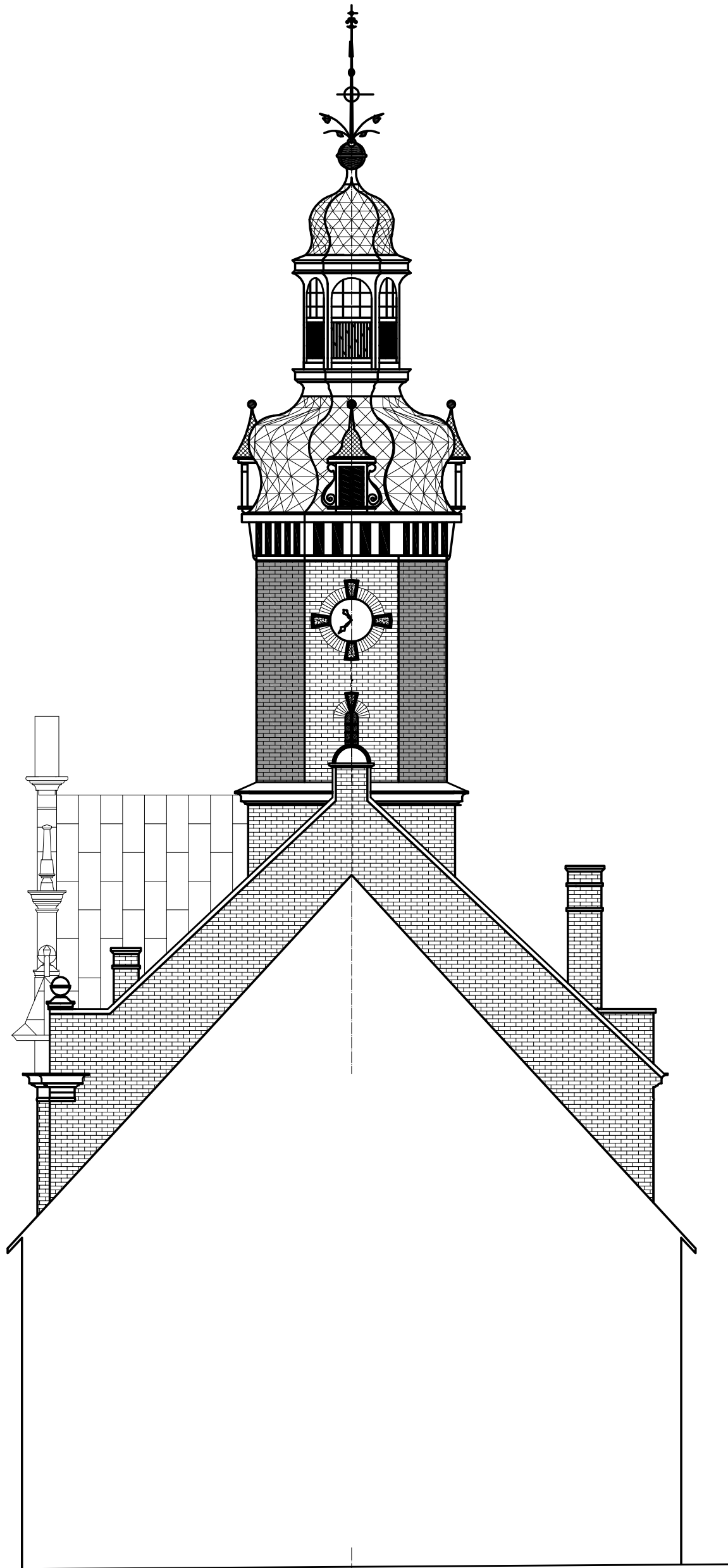
ELEWACJA POŁUDNIOWA - SKALA 1:100
