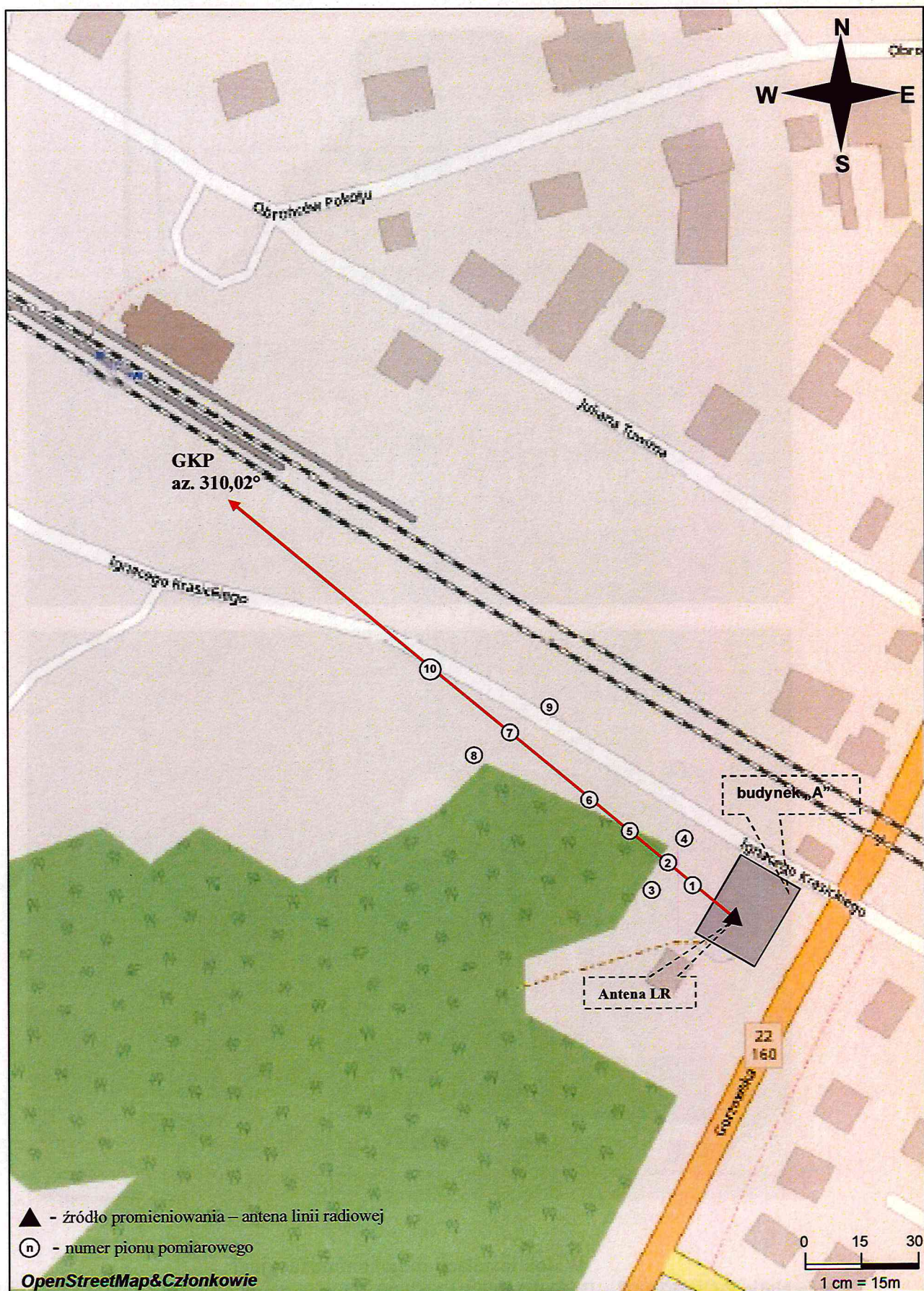
Rys. 1. Usytuowanie punktów i pionów pomiarowych w otoczeniu instalacji radiokomunikacyjnej Stacja Netia DOBWB008-DOBWM00001ANT001 Dobiegniew, ul. Leśna 2, nr działki 141/11 obręb Dobiegniew
